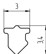
Уплотнитель ТПУ-65.07
